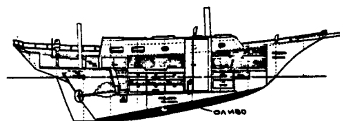
РИС.12 БАЛЯСТОВАНИЙ ВІТРИЛЬНИК
